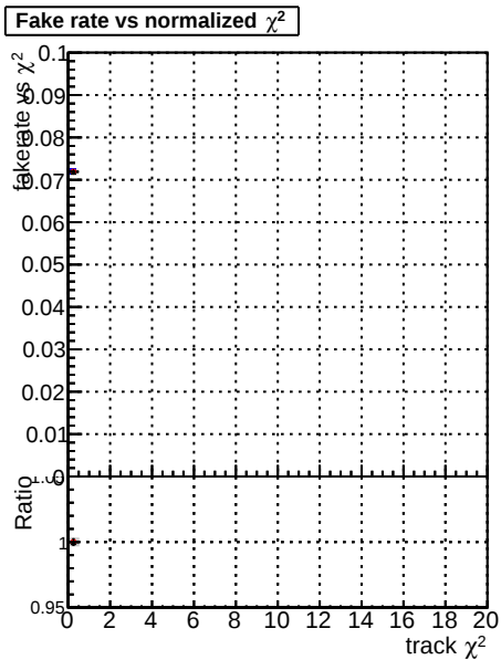
Fake rate vs. DOM CKF TTbarPU DOM mktT TTbarPU DOM mktT TTbarPU-clonerfix
