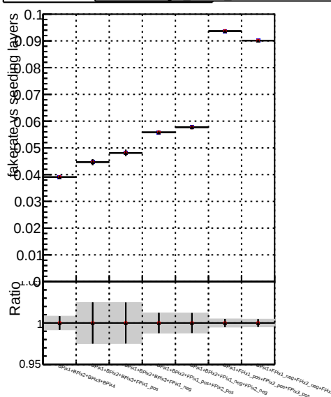
Fake rate vs. DOM CKF TTbarPU DOM mktT TTbarPU DOM mktT TTbarPU-clonerfix
