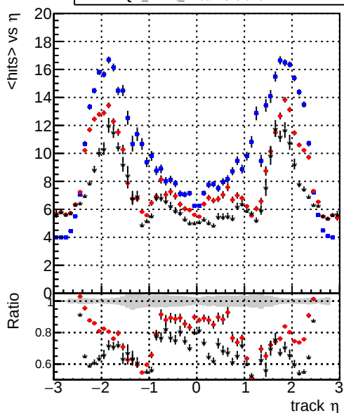
— DQM_CKF_TTbarPU — DQM_mkFit_TTbarPU — DQM_mkFit_TTbarPU-clonerfix
