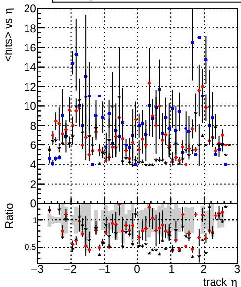
— DQM_CKF_TTbarPU — DQM_mkFit_TTbarPU — DQM_mkFit_TTbarPU-clonerfix mean hit
