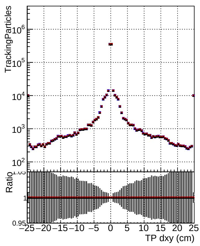
N of simulated track DQM_CKF_SoftQCD DQM_mkFit_SoftQCD- DQM_mkFit_SoftQCD-fixCloner
