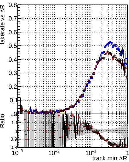
Legend: DOM_CKF_SoftQCD, DOM_mkFit_SoftQCD, DOM_mkFit_SoftQCD-fixCloner
