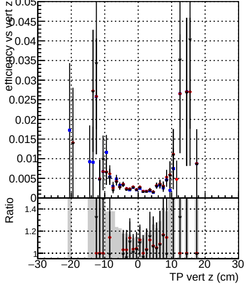
Efficiency vs vert z —●— DQM_CKF_SoftQCD —●— DQM_mkFit_SoftQCD- —●— DQM_mkFit_SoftQCD-fixCloner
