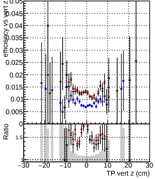
Efficiency vs. sim PV z — DQM_CKF_SoftQCD — DQM_mkFit_SoftQCD- — DQM_mkFit_SoftQCD-fixCloner
