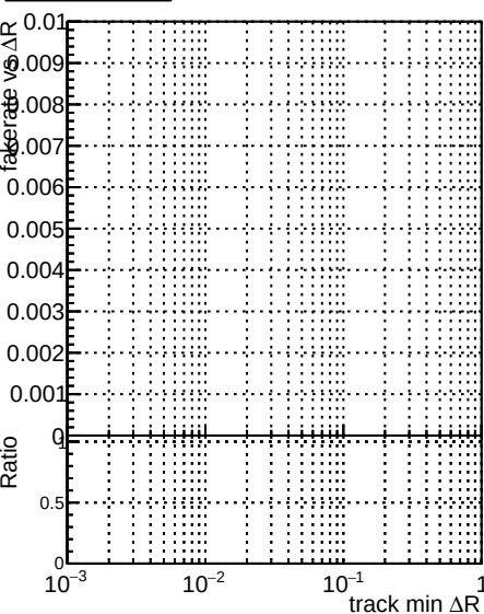
Fake rate vs \Delta R(\text{track, jet}) Legend: DQM_CKF_SoftQCD DQM_mkFit_SoftQCD DQM_mkFit_SoftQCD-fixCloner
