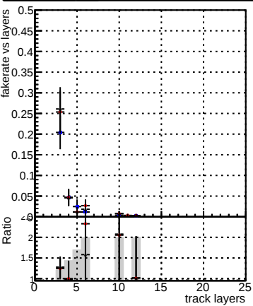
Fake rate vs hit Legend: DQM_CKF_SoftQCD DQM_mkFit_SoftQCD DQM_mkFit_SoftQCD-fixCloner
