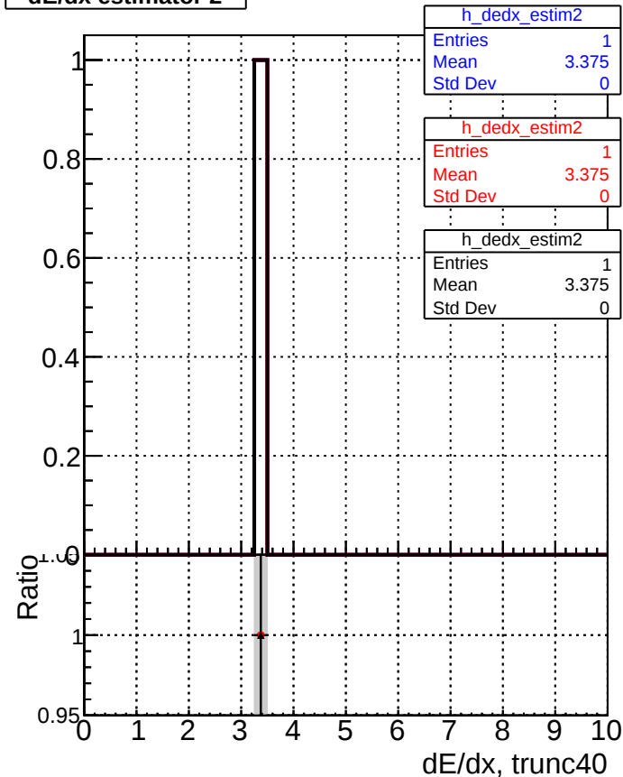
dE/dx estimator 2
