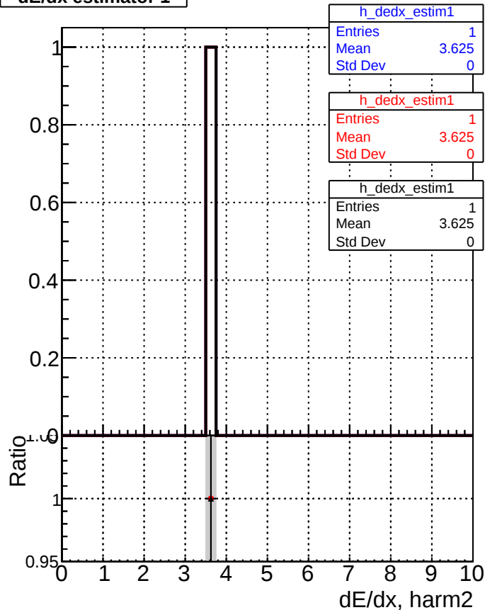
dE/dx estimator 1
