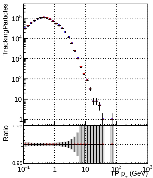
—•— DQM_CKF_SoftQCD —•— DQM_mkFit_SoftQCD- —•— DQM_mkFit_SoftQCD-fixCloner
