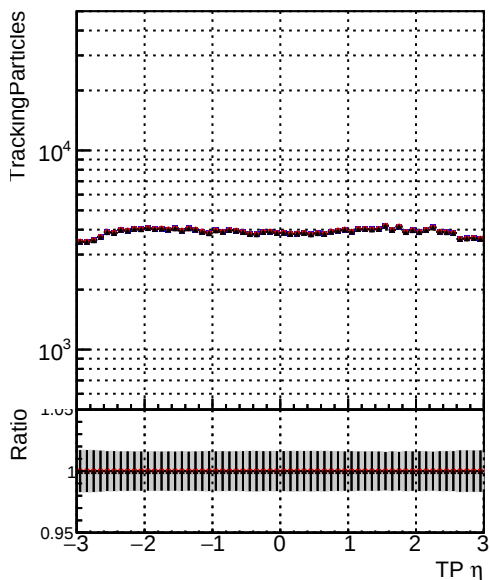
—•— DQM_CKF_SoftQCD —•— DQM_mkFit_SoftQCD- —•— DQM_mkFit_SoftQCD-fixCloner
