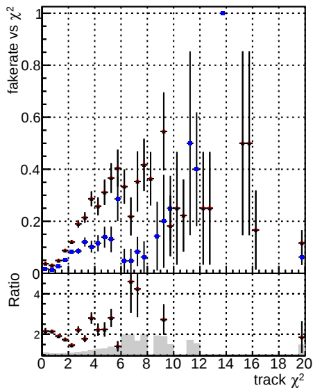
Fake rate vs. DOM CKF TTbar DOM mkt TTbar-newTr2
