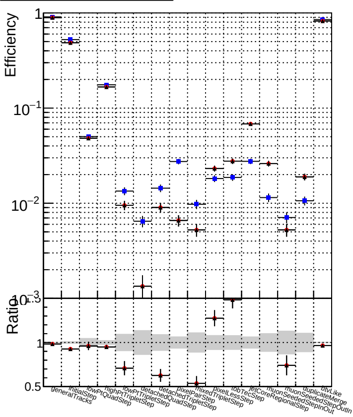
DQM_CKF_TTbar DQM_mkFit_TTbar DQM_mkFit_TTbar-newTr2
