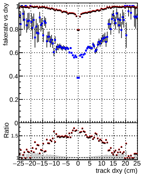
DOM CKE TTbar DOM mktT TTbar-newTr2
