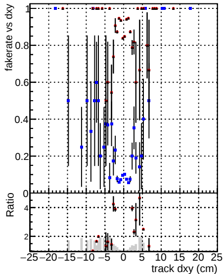
— DOM CKE T\bar{T} bar — DOM mkt T\bar{T} bar — DOM mkt T\bar{T} bar-newTr
