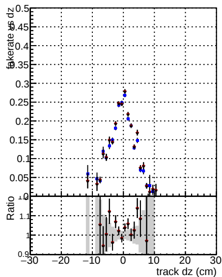
DOM CKF TTbar DOM CKF TTbarPU-ncp DOM CKF TTbarPU-newTr6
