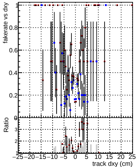
— DOM CKE T\bar{T} bar — DOM mktFit T\bar{T} bar — DOM PU-nep
