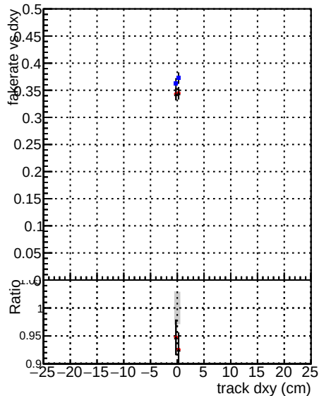
— DOM CKF TTbar — PU-ncp — DOM mkFit TTbar PU-newTr5
