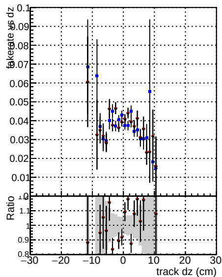
—•— DOM CKF TTbar —•— DOM CKF TTbarPU-ncp —•— DOM CKF TTbarPU-newTr5
