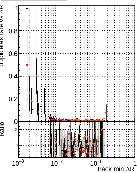
Legend: DOM, CKF, TTbar, mktFit, TTbar, PU-ncp, PU-newTr4
