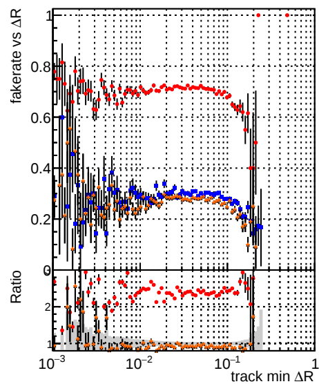
Fake rate vs \Delta R(\text{track, jet}) Legend: DQM CKE TTbar DQM mktFit TTbar DQM mktFit TTbar PU-ncp DQM mktFit TTbar PU-newTr4
