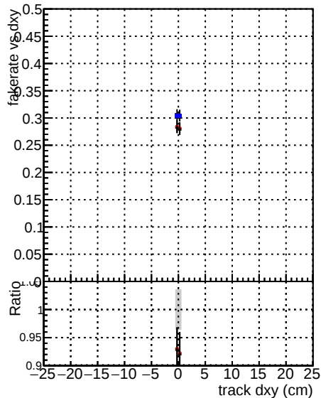
— DOM CKF TTbar — DOM CKF TTbarPU-ncp — DOM CKF TTbarPU-newTr4
