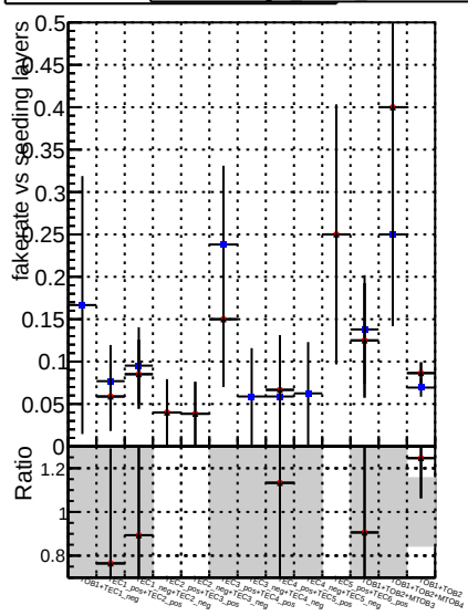
Fake rate vs. DOM CKE TTbar DOM mktT TTbarPU-nep DOM mktT TTbarPU-newTr4
