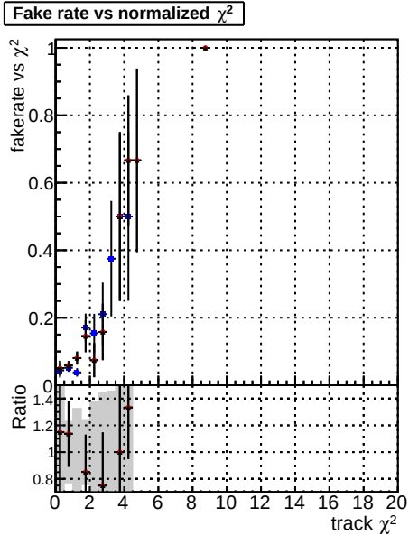
Fake rate vs. DOM CKE TTbar DOM mktT TTbarPU-nep DOM mktT TTbarPU-newTr4
