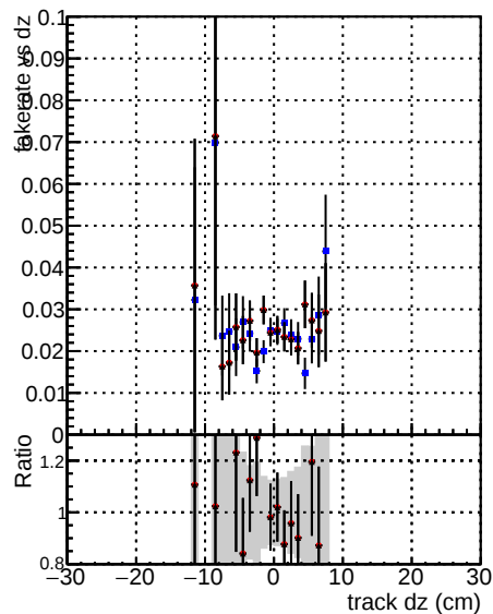
— DOM CKF TTbar — BQM mktFit TTbarPU-ncp — BQM mktFit TTbarPU-newTr4
