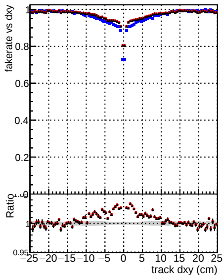
— DOM CKF T\bar{T} bar — DOM mkt T\bar{T} barPU-ncp — DOM mkt T\bar{T} barPU-newTr4
