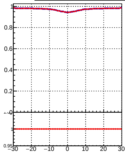
■ DQM_Original —●— DQM_Modified
