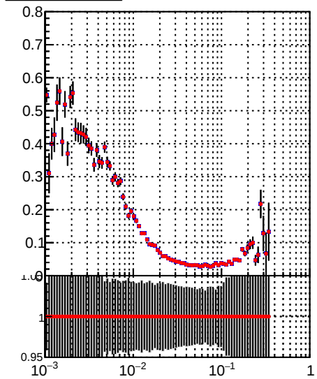
Fake rate vs \sqrt{s} DQM_Original DQM_Modified
