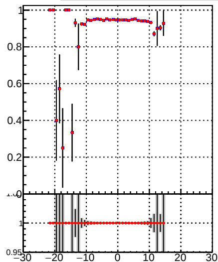
■ DQM_Original ◆ DQM_Modified
