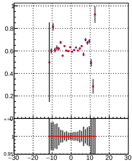
Fake rate vs \Delta y
