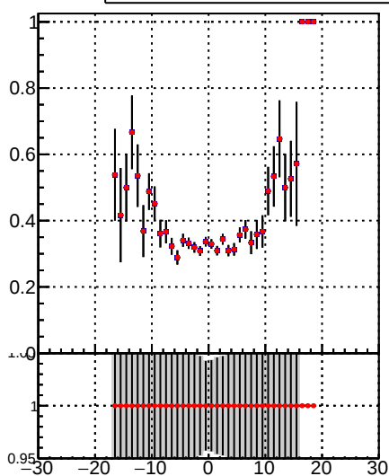
DQM_Original DQM_Modified
