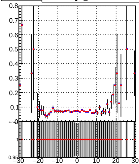
█ DQM_Original ● DQM_Modified
