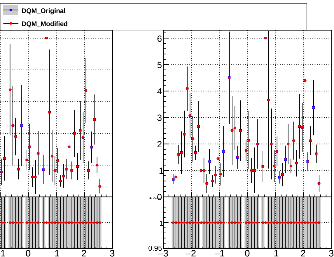
mean # STRIP hits vs eta
