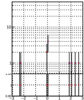
pT [GeV]
