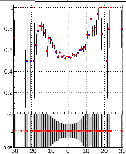
DQM_Original DQM_Modified
