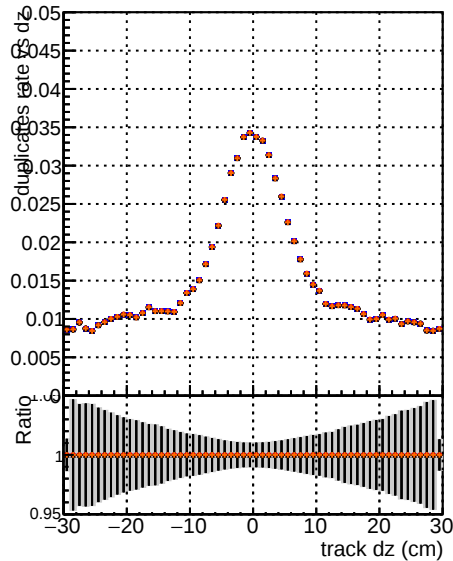
CNN
