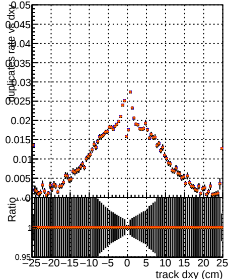
CNN
