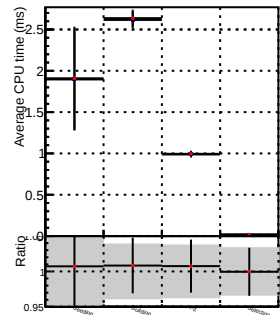
muonSeededSteps
