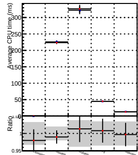
tobTecStep
