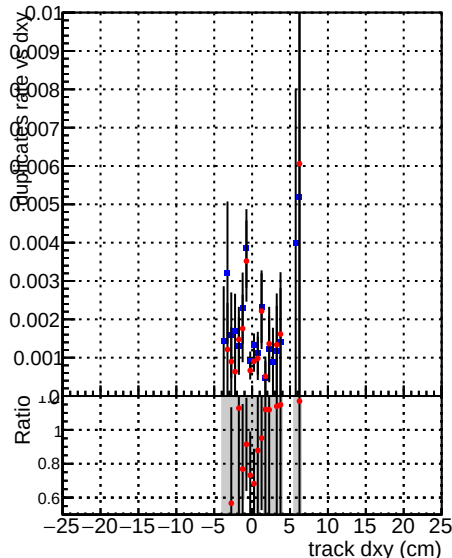
—■— DQM V0001 R0000000001 Global mkFit1000i0 RECO —●— DQM V0001 R0000000001 Global mkFit1000mod RECO
