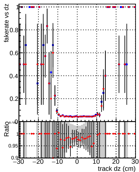
— Global mkFitQCDi1 RECO — Global mkFitQCDmod RECO
