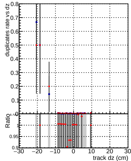
— Global mkFitQCDi1 RECO — Global mkFitQCDmod RECO
