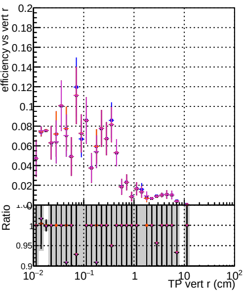
Efficiency vs TP vert r (cm) DOM CKFit-test 1000evt DOM mkFitREFit-test 1000evt DOM mkFitREFit-OR-test 1000evt DOM mkFitREFit-ORK-test 1000evt DOM mkFitREFit-OR4-test 1000evt
