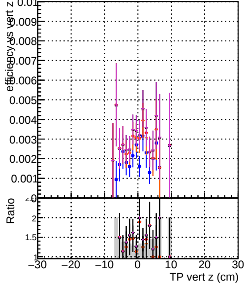
Efficiency vs vert z — DOM CKFit-test_1000evt — DOM mkFitREFit-test_1000evt — DOM mkFitREFit-ORk-test_1000evt — DOM mkFitREFit-OR4-test_1000evt
