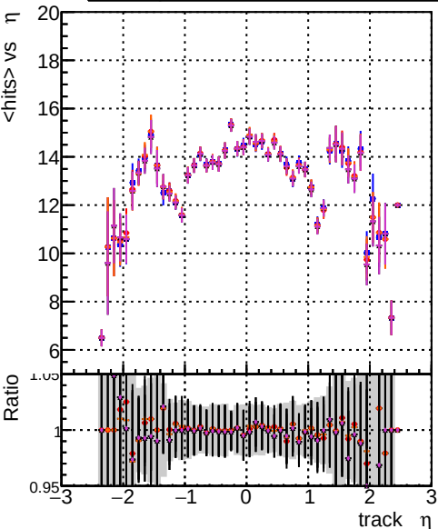
mean hits vs \eta DOM CKF-test 1000evt DOM mkFitREFit-test 1000evt DOM mkFitREFit-OR4-test 1000evt DOM mkFitREFit-test 1000evt
