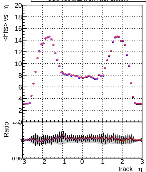
mean hits vs \eta DOM CKFit-test 1000evt DOM mkFitREFit-test 1000evt DOM mkFitREFit-OR4-test 1000evt DOM mkFitREFit-OR4-test 1000evt
