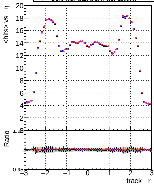
mean hits vs \eta DOM CKFit-test 1000evt DOM mkFitREFit-test 1000evt DOM mkFitREFit-OR4-test 1000evt DOM mkFitREFit-test 1000evt DOM mkFitREFit-OR4-test 1000evt
