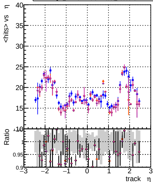
mean hits vs \eta DOM CKFit-test 1000evt DOM mkFitREFit-test 1000evt DOM mkFitREFit-OR-test 1000evt DOM mkFitREFit-ORK-test 1000evt DOM mkFitREFit-OR4-test 1000evt
