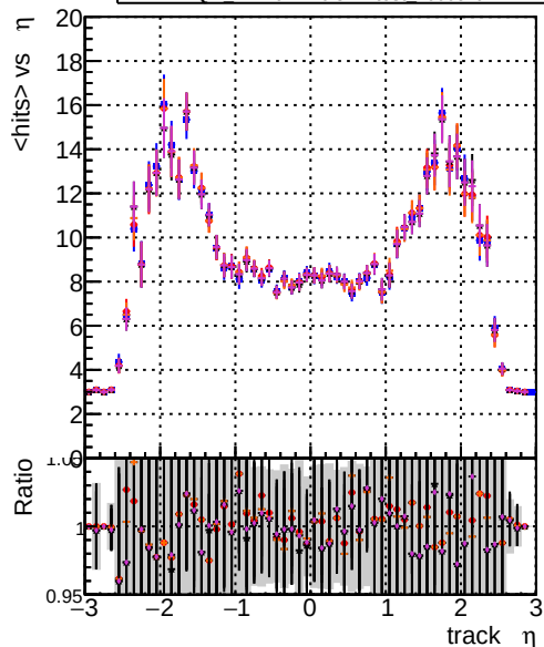
mean hits DOM CKFit-test 1000evt DOM mkFitREFit-test 1000evt DOM mkFitREFit-OR4-test 1000evt DOM mkFitREFit-test 1000evt
