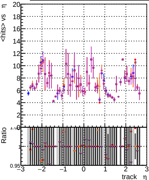
mean hits vs \eta DOM CKFit-test 1000evt DOM mktFitREFit-test 1000evt DOM mktFitREFit-OR4-test 1000evt DOM mktFitREFit-OR4-test 1000evt
