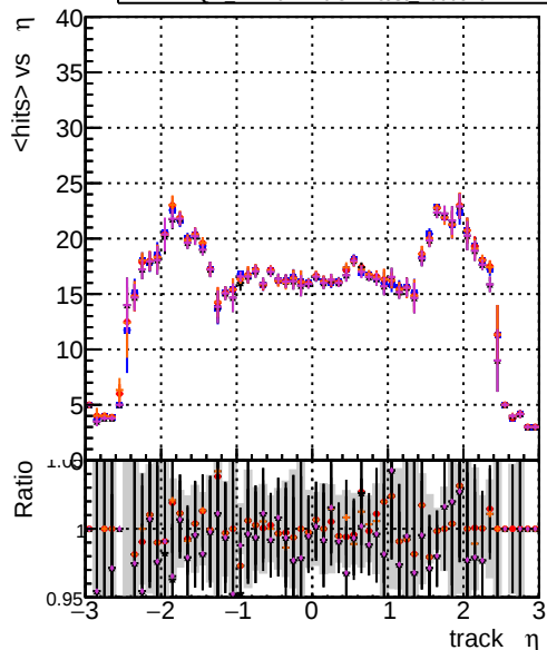
mean hits vs \eta DOM CKFit-test 1000evt DOM mkFitREFit-test 1000evt DOM mkFitREFit-OR4-test 1000evt DOM mkFitREFit-test 1000evt
