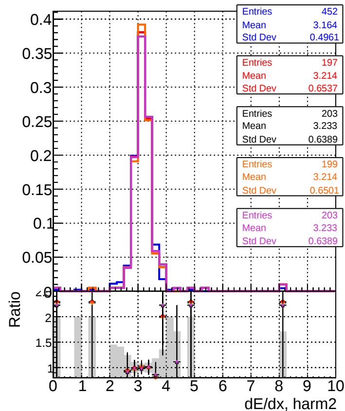
DOM_CKF-test_1000evt DOM_mkFitREFit-test_1000evt DOM_mkFitREFit-OR-test_1000evt DOM_mkFitREFit-ORK-test_1000evt DOM_mkFitREFit-OR4-test_1000evt
