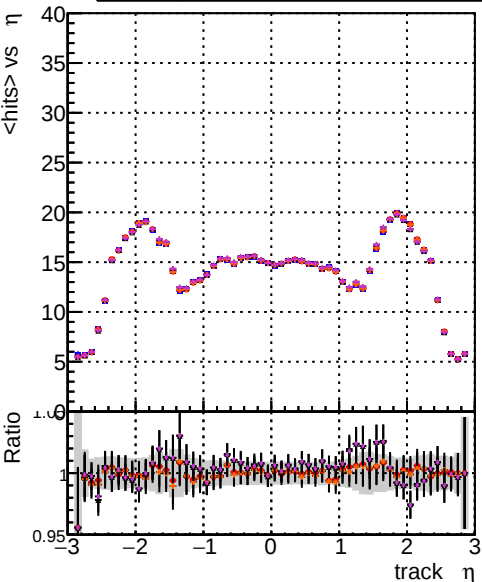
mean hits vs \eta DOM CKF-test_1000evt DOM mkFitREFit-test_1000evt DOM mkFitREFit-OR-test_1000evt DOM mkFitREFit-ORK-test_1000evt DOM mkFitREFit-OR4-test_1000evt
