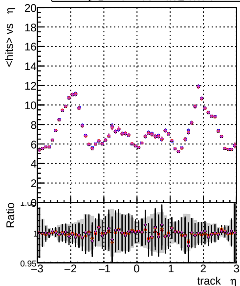
mean hits vs \eta DOM CKF-test 1000evt DOM mkFitREFit-test 1000evt DOM mkFitREFit-OR4-test 1000evt DOM mkFitREFit-OR4-test 1000evt
